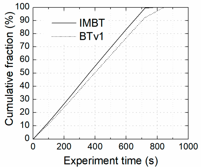
(d) CDFs of completion time (swarm size is 300)
